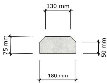
COPING TYPE 8 (180)
